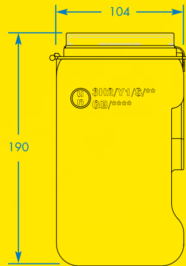
VUE LATÉRALE
